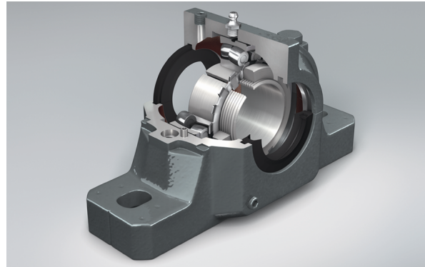
↑ SNN-Lagergehäusen mit Hochleistungs-Pendelrollenlagern und Labyrinthdichtungen
